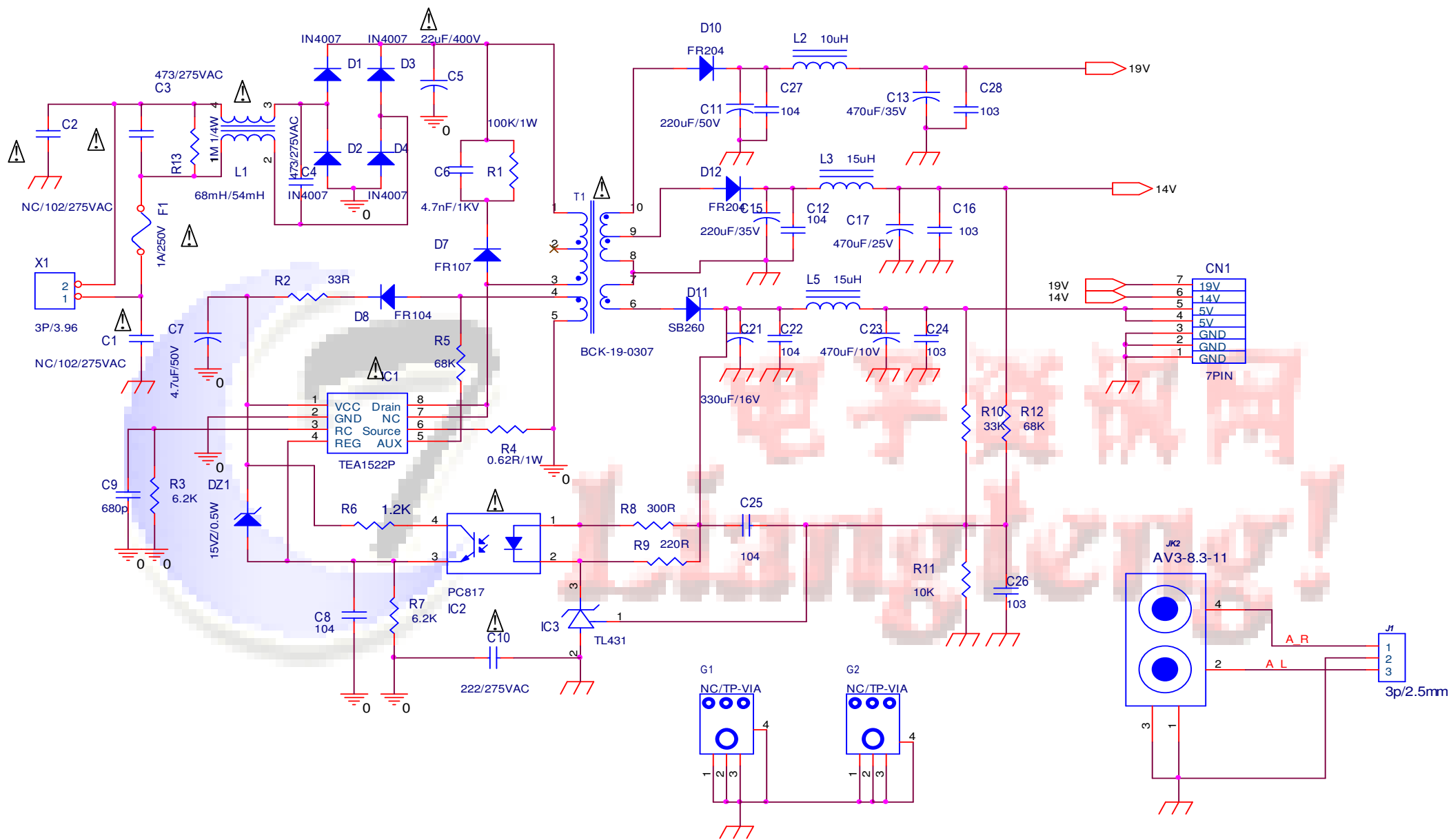
TEA1522p 电源板电路图，用于 DVB-S 机顶盒内，输入 80~250V，输出 19V，14V，5V。
